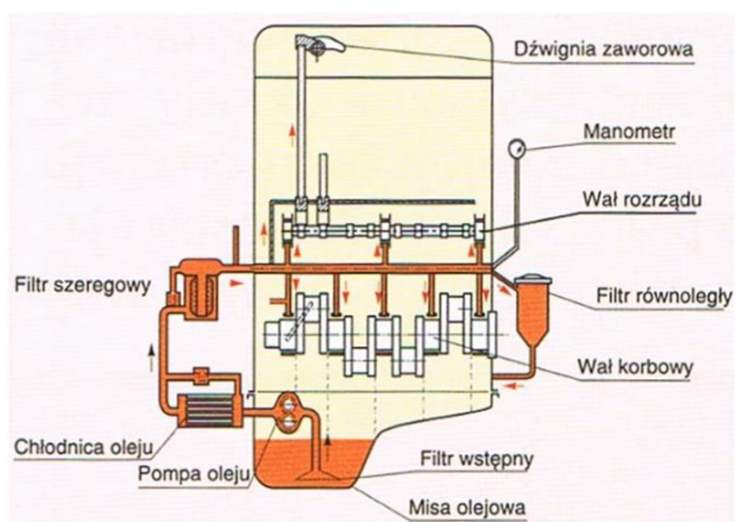
Schemat układu smarowania pod ciśnieniem
